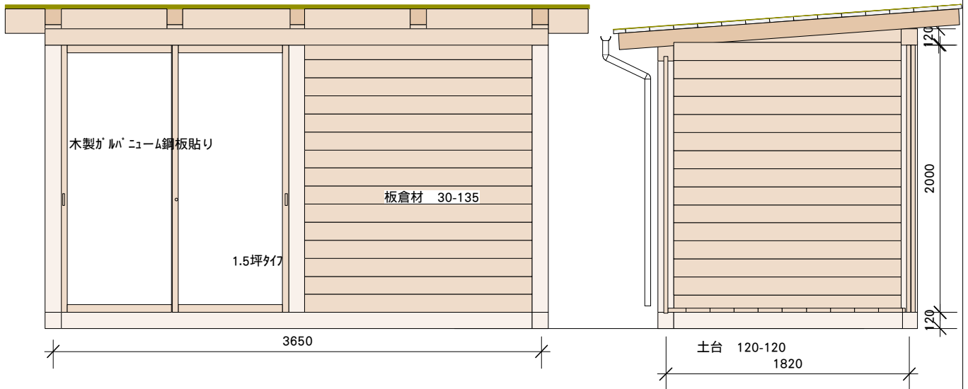
立面図
