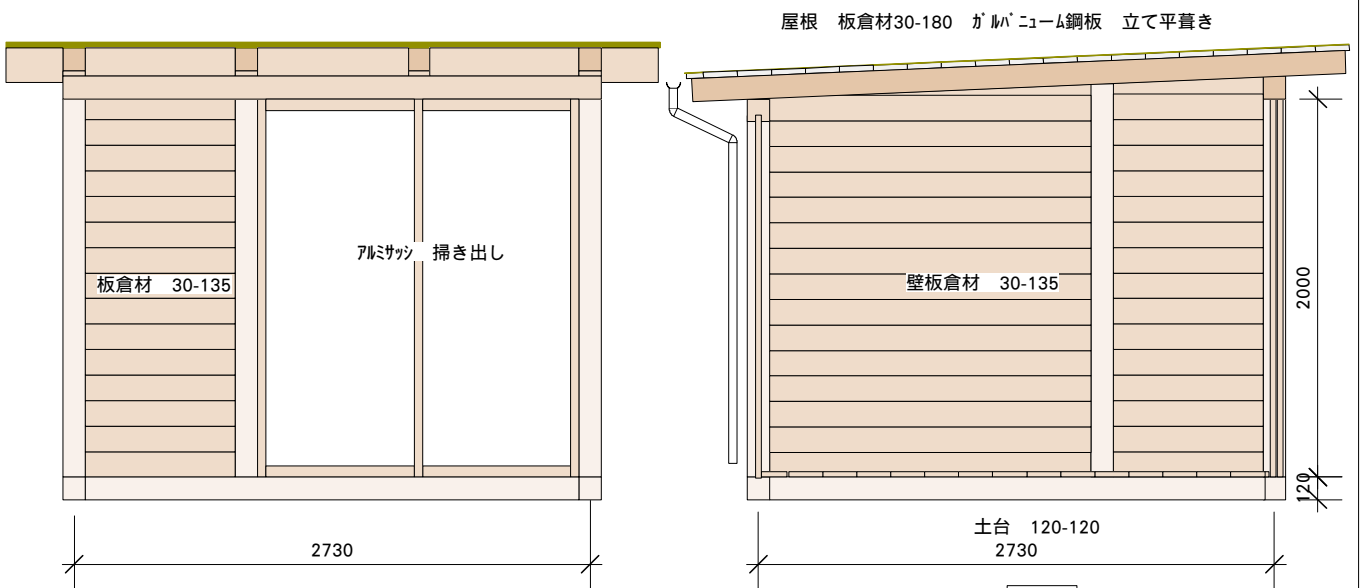
立面図
