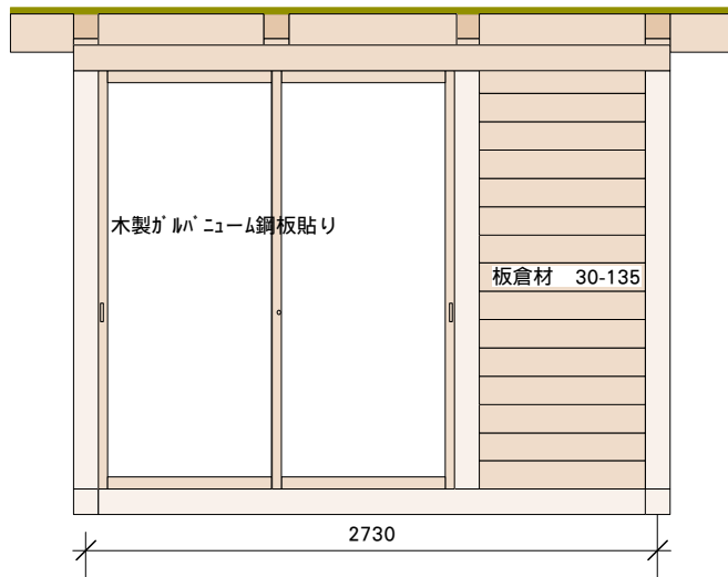
立面図
