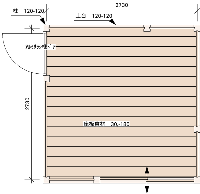
平面図
