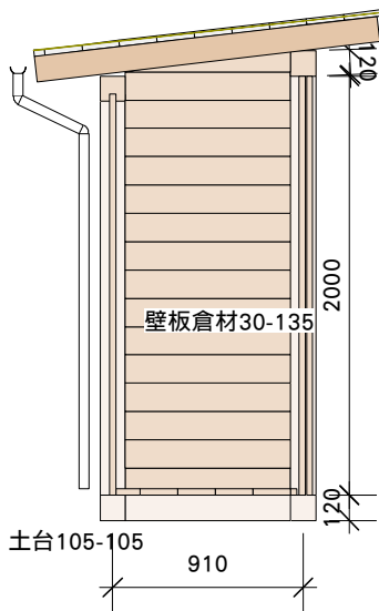
断面図
