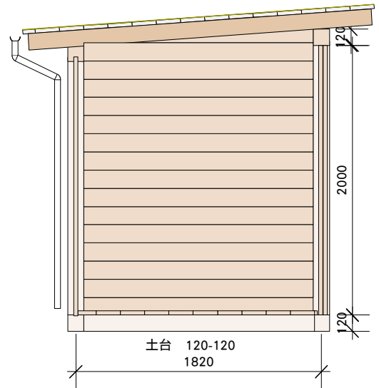
断面図
