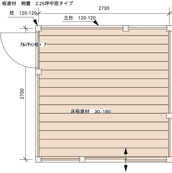
平面図
