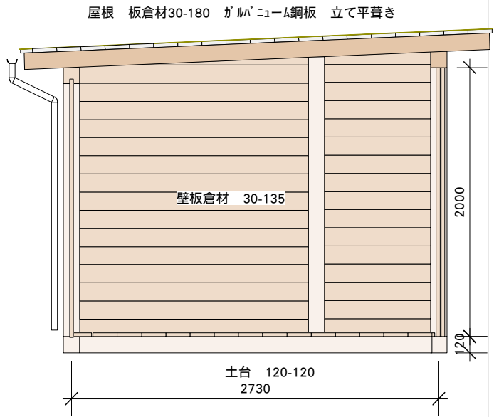
断面図
