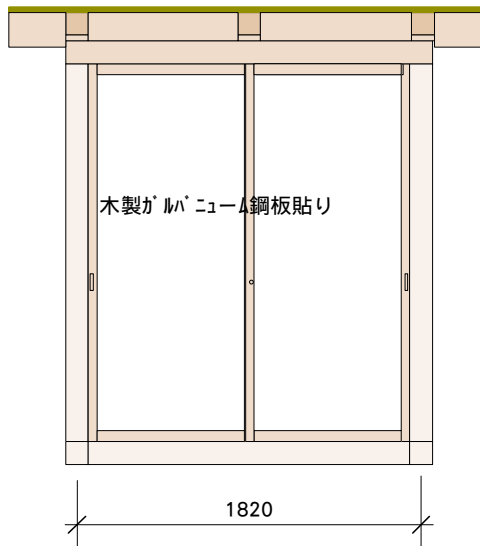
立面図
